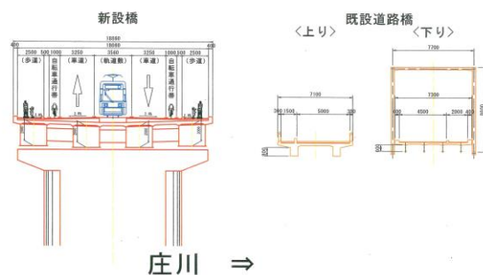
新庄川橋 標準横断面図 S=1:200
